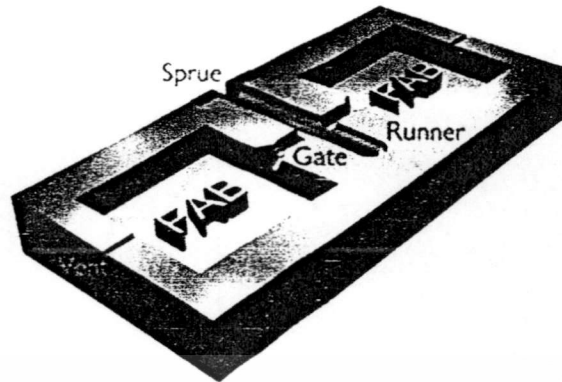
รูปที่ 3.36 ทางเข้าและระบบป้อน [1]
