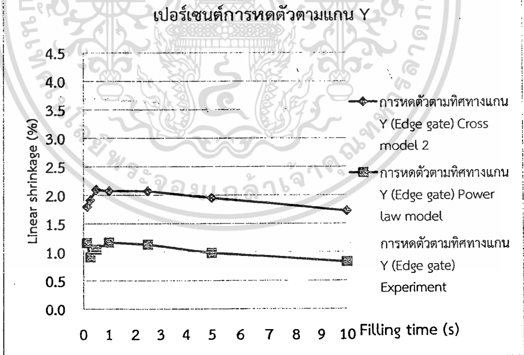
รูปที่ 5.30 ค่าการหดตัวเฉลี่ยของชิ้นงานในทิศทางตามการไหล ตามแกน Y ของชิ้นงาน Edge gate
