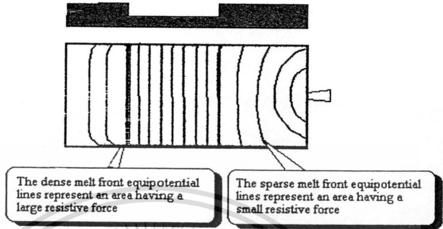
รูปที่ 3.14 ลักษณะเคลื่อนตัวของพลาสติกเหลว Melt front ผ่านแม่พิมพ์ที่หนาแตกต่างกัน [1]
