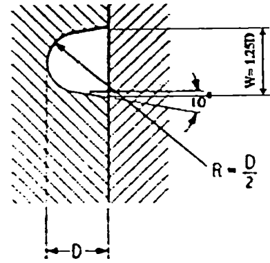
รูปที่ 3.34 ทางวึ่งหน้าตัดรูป Parabolic [19]
