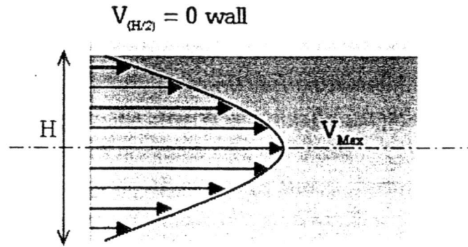
รูปที่ 3.16 รูปแบบการไหลที่เกิดความแตกต่างของความดันภายในช่องทางการไหลพื้นที่หน้าตัดสี่เหลี่ยม [1]
