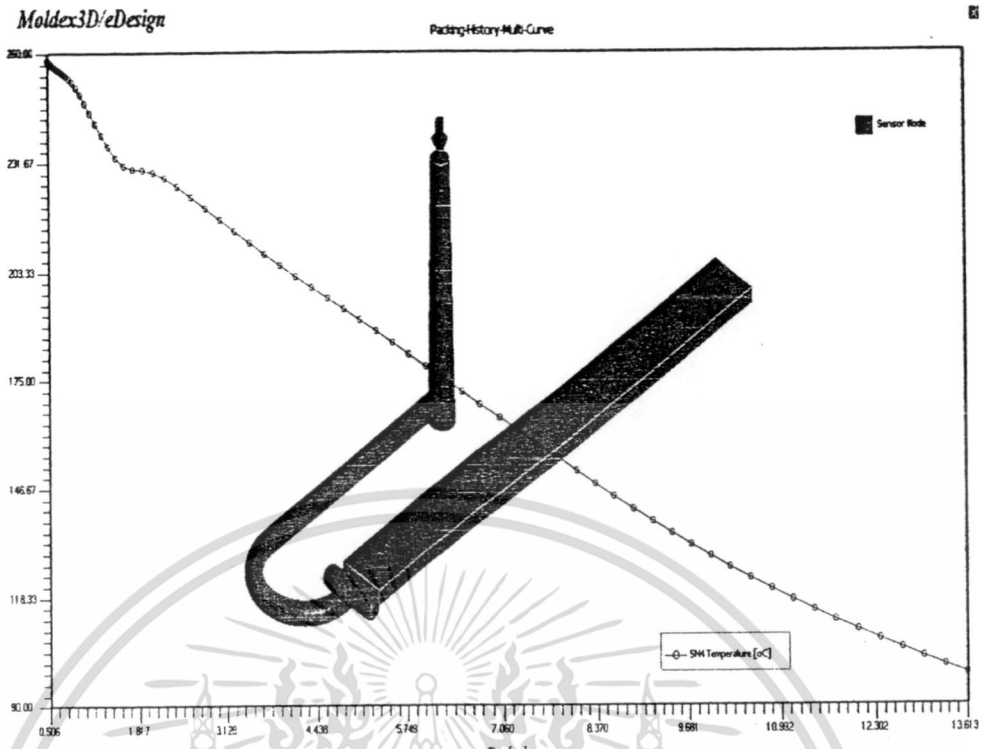
รูปที่ 5.32 อุณหภูมิที่เวลาในการฉีดย่ำที่ทางเข้าของชิ้นงานแบบ Film gate ที่ 0.5 วินาที
