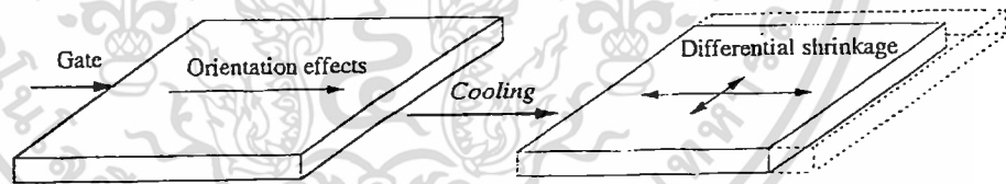
รูปที่ 2.19 พฤติกรรมการหดตัวในทิศทางการไหลและทิศทางตั้งฉากการไหล [33]
