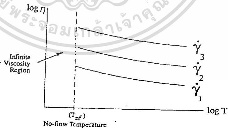
รูปที่ 3.24 ข้อมูลของความหนืดกับเส้นยุติการไหล
