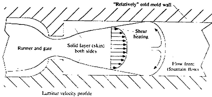
รูปที่ 3.12 การเย็นตัวอย่างรวดเร็วที่ผนังแม่พิมพ์ ที่เกิดจากอุณหภูมิผนังโพรงแบบเย็น [7]
