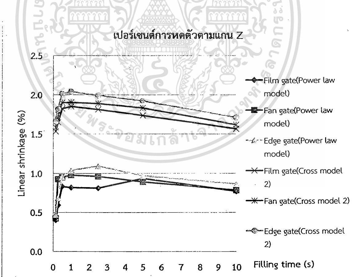
รูปที่ 5.22 ค่าการหดตัวเฉลี่ยของชิ้นงานในทิศทางตั้งฉากการไหล ตามแกน Z
