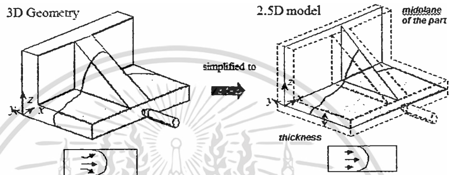
รูปที่ 2.7 พฤติกรรมการไหลของชิ้นงาน 3D (ซ้าย) และชิ้นงาน 2.5D midplane (ขวา) [1]
