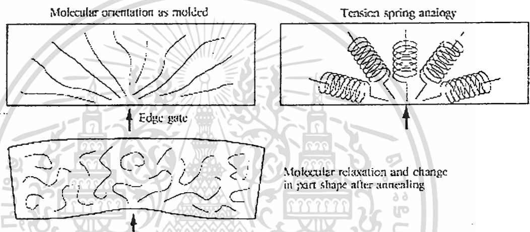
รูปที่ 3.11 พฤติกรรมการหดตัวกลับของสายโซ่โพลิเมอร์หลังจากทางเข้าเย็นตัว [7]
