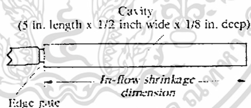
รูปที่ 2.15 ชิ้นงานตามมาตรฐาน ASTM D955-08 [33]
