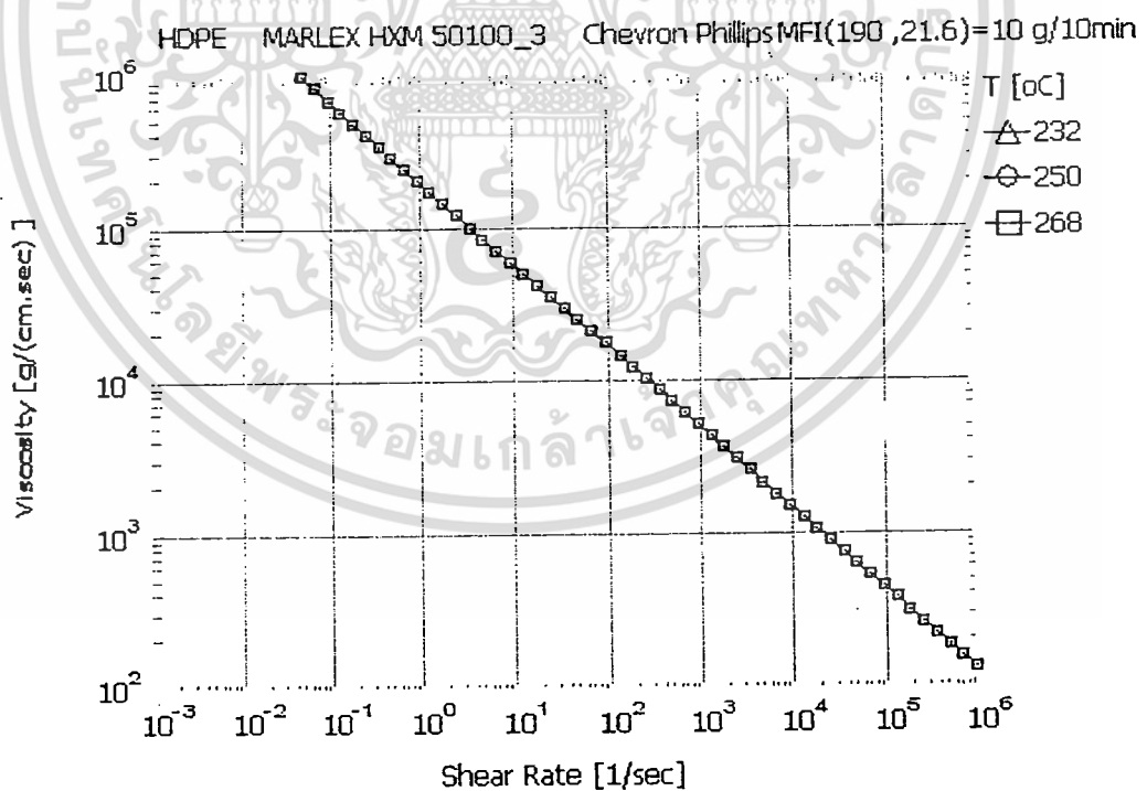
รูปที่ 5.8 ความสัมพันธ์ระหว่างอัตราเฉือนและความหนืด Power law model
