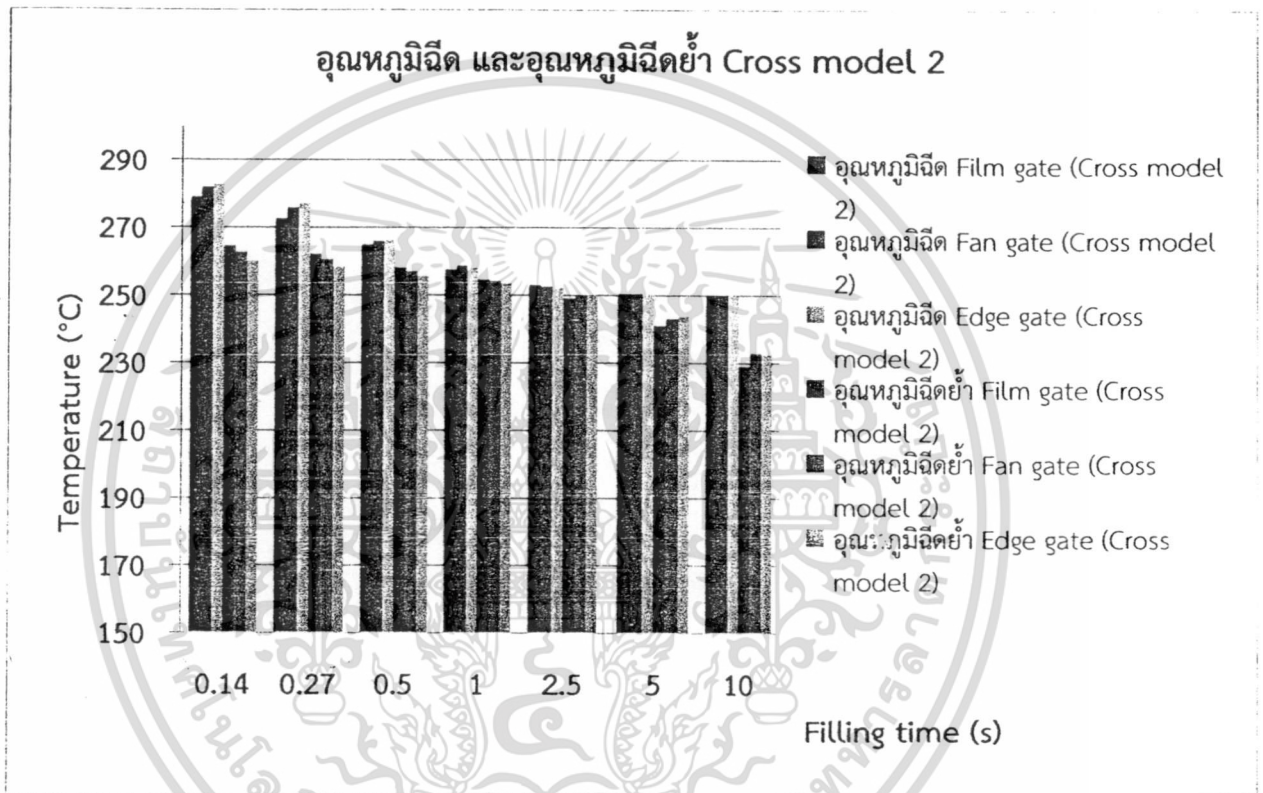
รูปที่ 5.12 อุณหภูมิฉีด และอุณหภูมิฉีดย้ำต่อเวลาฉีด (Cross model 2)
