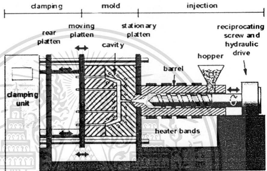
รูปที่ 3.28 องค์ประกอบของกระบวนการฉีดพลาสติก [5]
