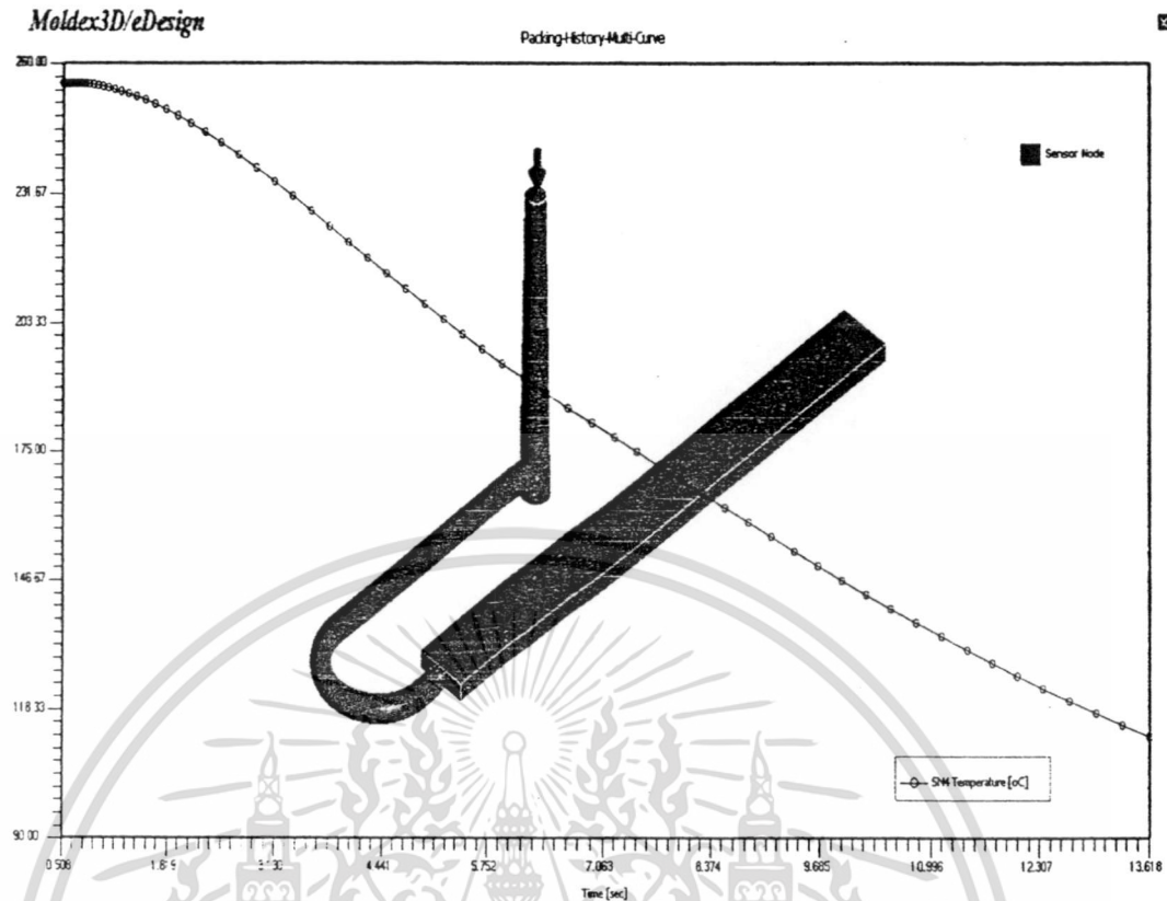
รูปที่ 5.34 อุณหภูมิที่เวลาในการฉีดที่ยังที่ทางเข้าของชิ้นงานแบบ Edge gate ที่ 0.5 วินาที
