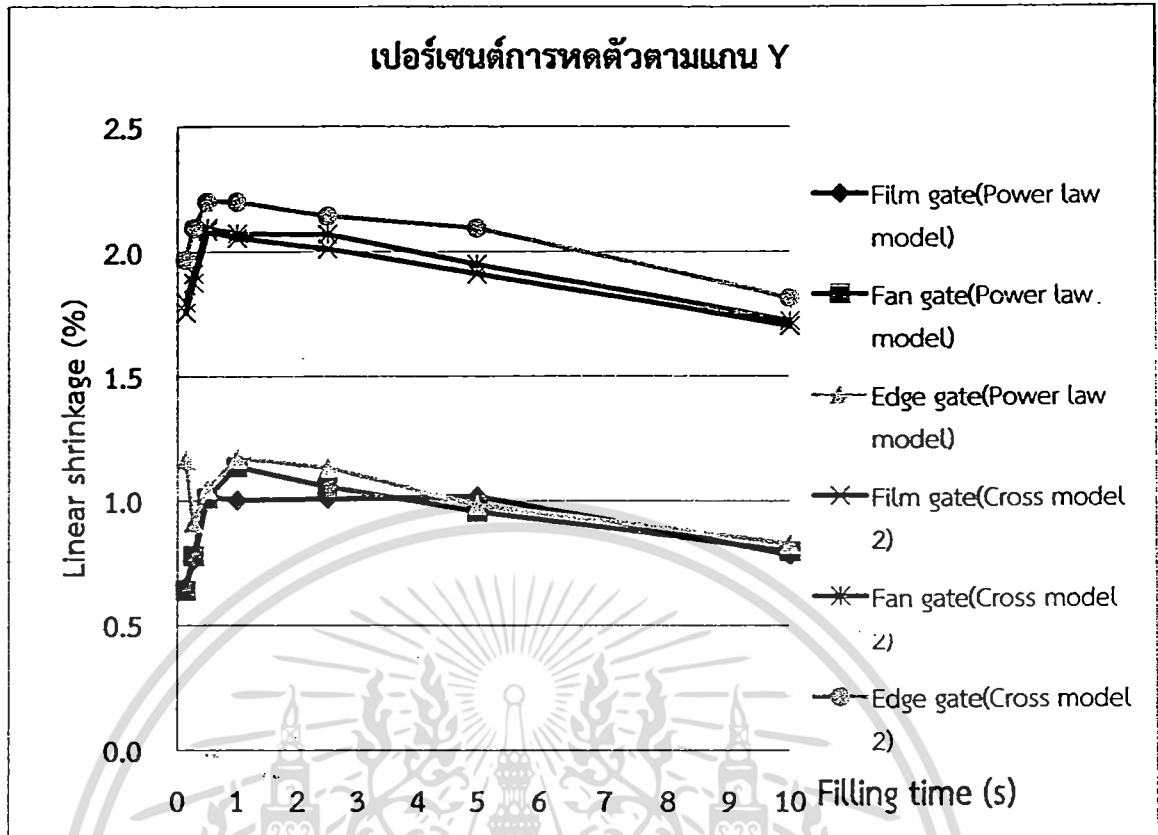
รูปที่ 5.21 ค่าการหดตัวเฉลี่ยของชิ้นงานในทิศทางตามการไหล ตามแกน Y
