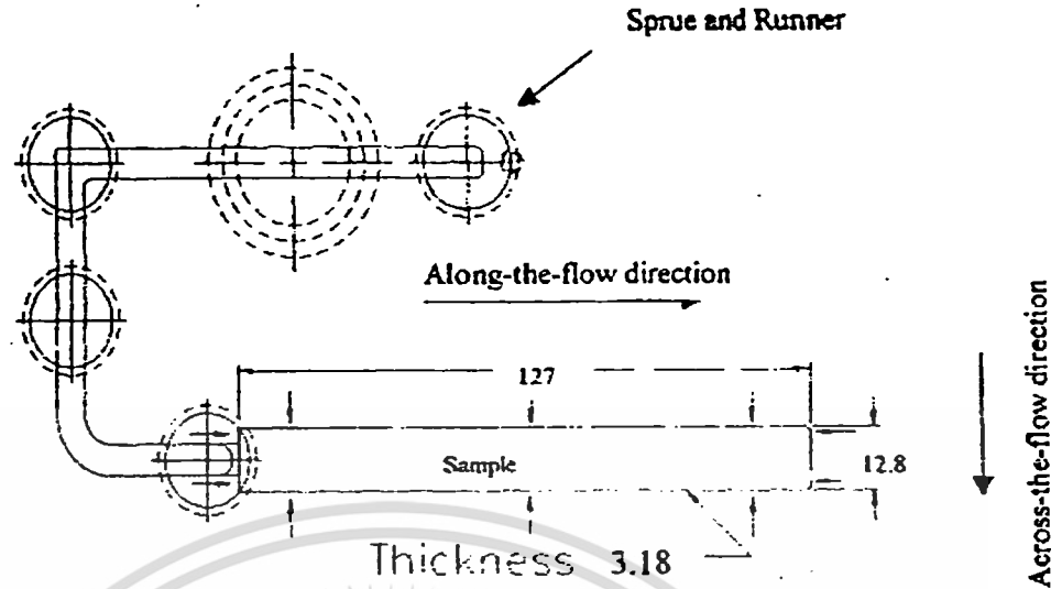
รูปที่ 2.16 โมเดลการทดสอบการหดตัว Chang (2003)
