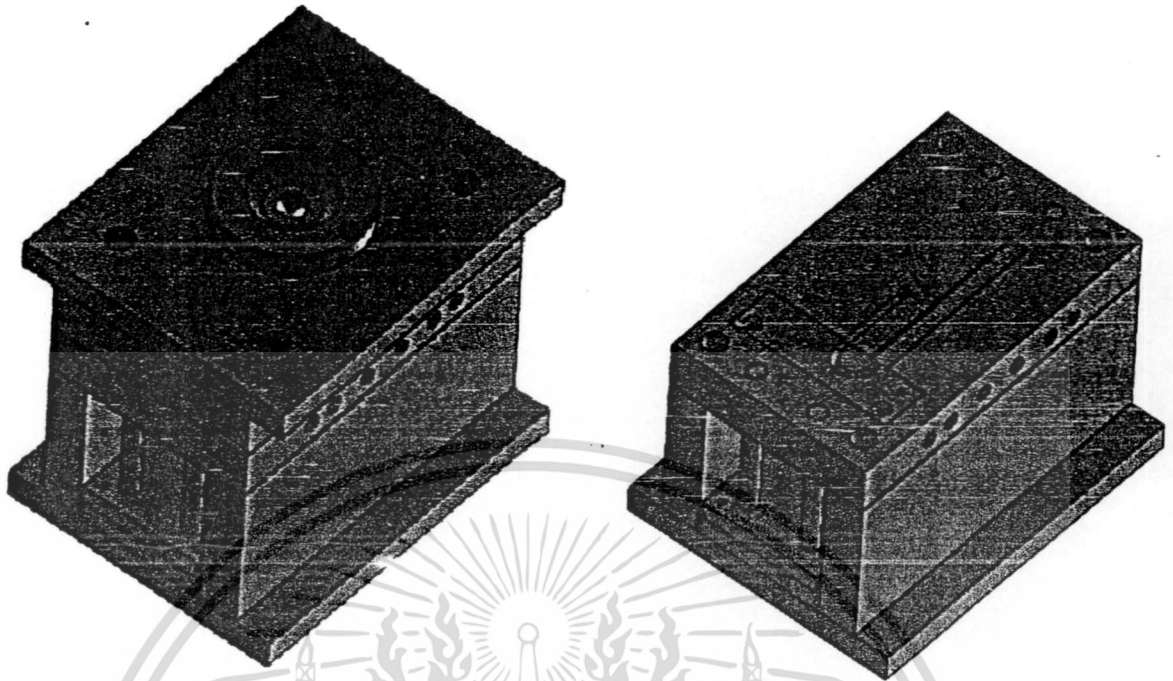
รูปที่ 5.4 ลักษณะแม่พิมพ์ฉีดขึ้นงานตามมาตรฐาน ASTM D955-08 (ซ้าย) และลักษณะโพรงแบบ (ขวา)
