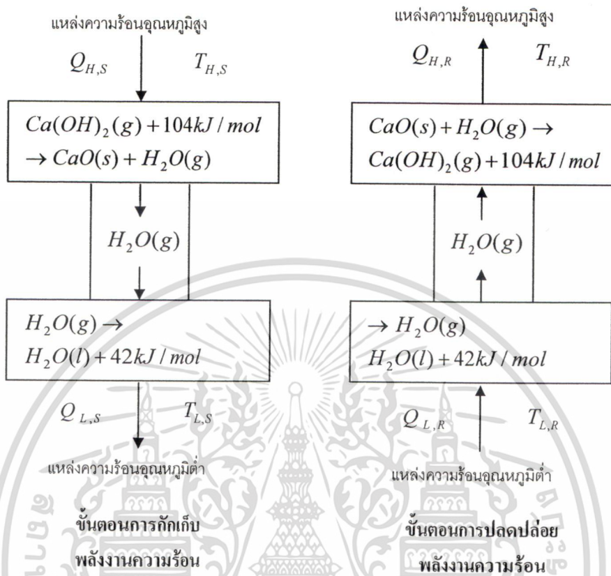
รูปที่ 2.6 การทำงานของปั๊มความร้อนพลังงานเคมีที่ให้แคลเซียมออกไซด์ และน้ำ ในการทำปฏิกิริยา ปรับปรุงจาก [1]
