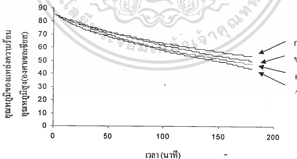
รูปที่ ก.1 ความสัมพันธ์ระหว่างอุณหภูมิของแหล่งความร้อนอุณหภูมิต่ำสูงกับเวลา
