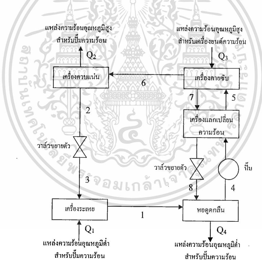
รูปที่ 2.3 ปั๊มความร้อนชนิดดูดกลืน ปรับปรุงจาก [2]
