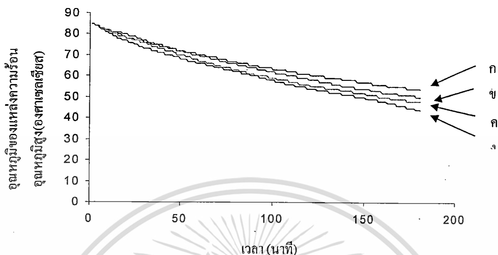
รูปที่ ข.1 ความสัมพันธ์ระหว่างอุณหภูมิของแหล่งความร้อนอุณหภูมิต่ำกับเวลา เมื่ออุณหภูมิของแหล่งความร้อนอุณหภูมิต่ำต่างกัน
