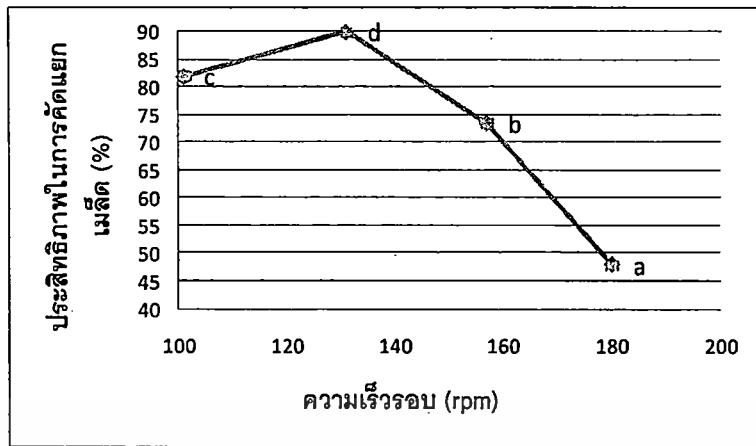
รูปที่ 4.7 ความสัมพันธ์ระหว่างความเร็วรอบและประสิทธิภาพการตัดแยกเมล็ด
