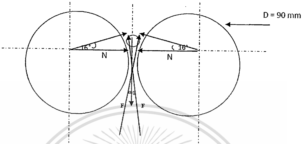
รูปที่ 3.4 ไตอะแกรมการรับแรงของเมล็ดสบู่ดำมีระยะห่างมากที่สุด 9 mm
