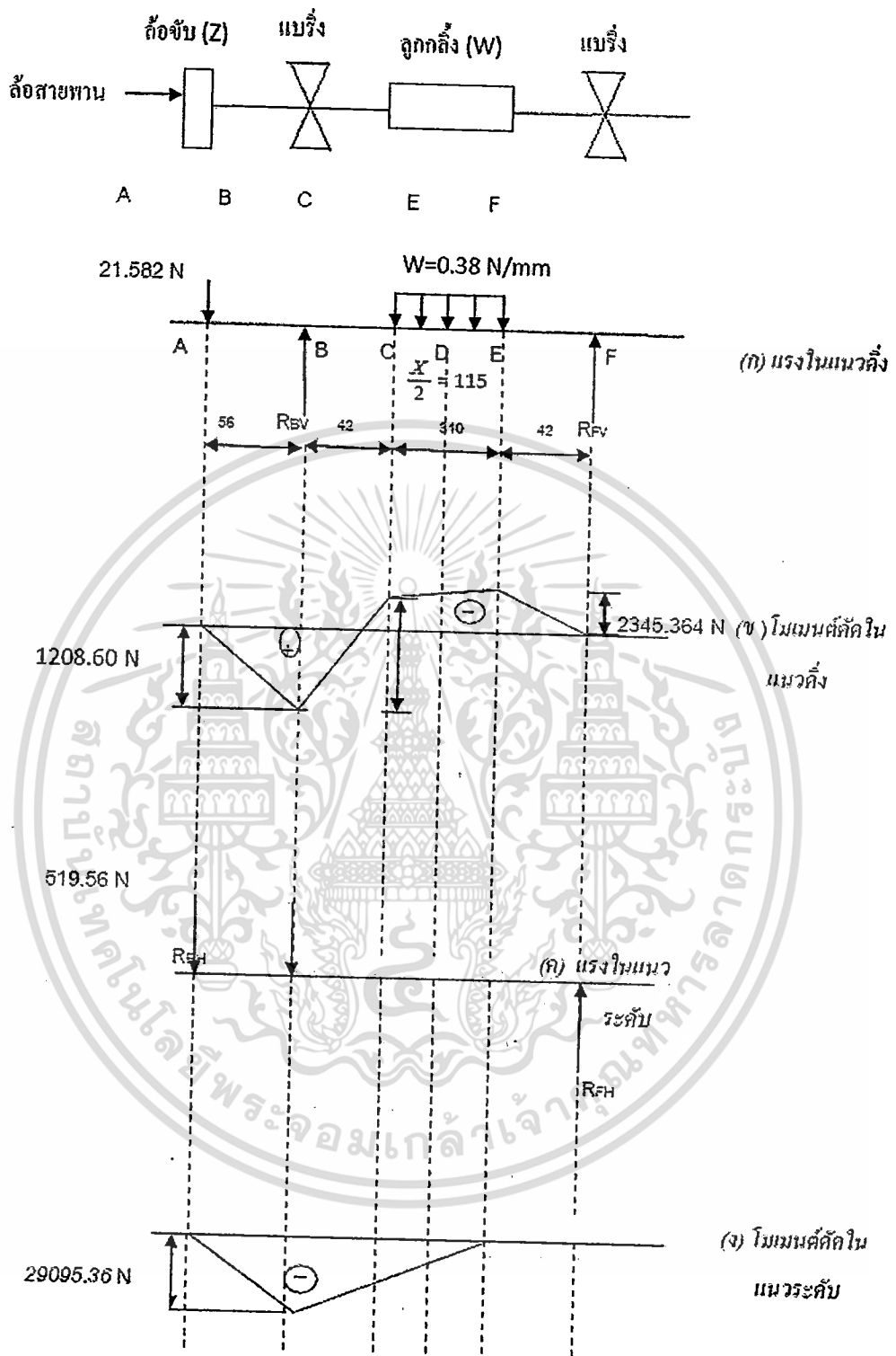
รูปที่ 3.9 กราฟแสดงแรงเฉือนและ โมเมนต์คัตที่เกิดดับเพลาลูกกลิ้งในแนวตั้ง
