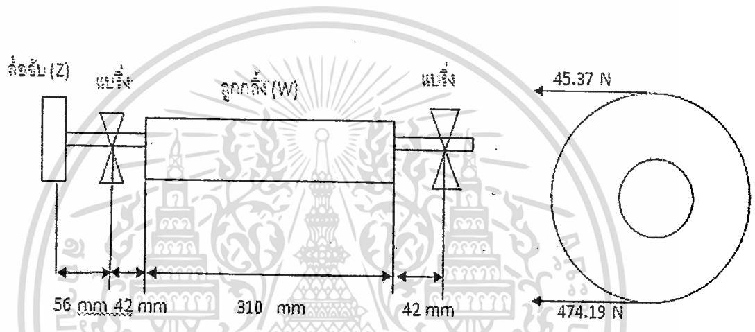
รูปที่ 3.8 ชิ้นส่วนต่างๆของชุดลูกกลิ้งที่มีแรงกระทำต่อเพลา
