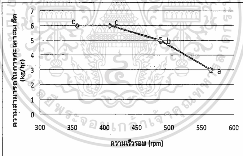
รูปที่ 4.10 ความสัมพันธ์ระหว่างความเร็วรอบและความสามารถในการกะเทาะเมทัลสบูดำ
