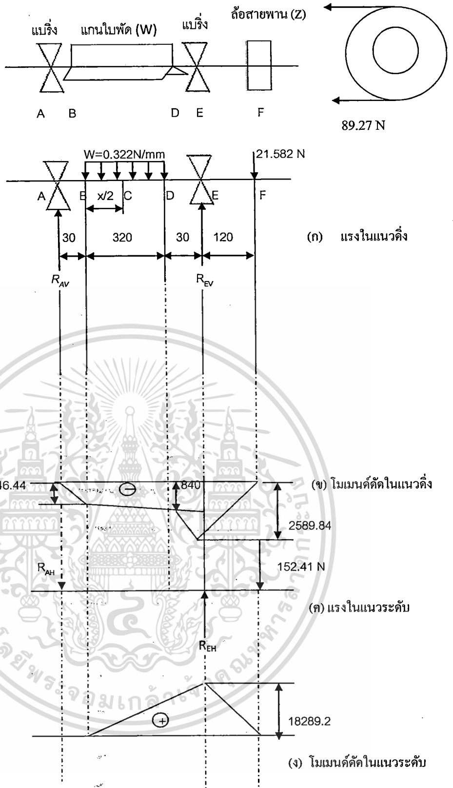
รูปที่ 3.10 กราฟแสดงแรงเฉือนและ โมเมนต์ค้ดที่เกิดกับเพลา โบลว์เวอร์
