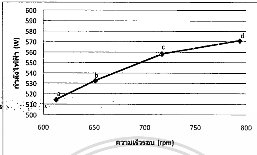
รูปที่ 4.14 ความสัมพันธ์ระหว่างความเร็วรอบและกำลังไฟฟ้าในการตัดแยกเปลือกเมล็ด ออกจากเนื้อในเมล็ด
