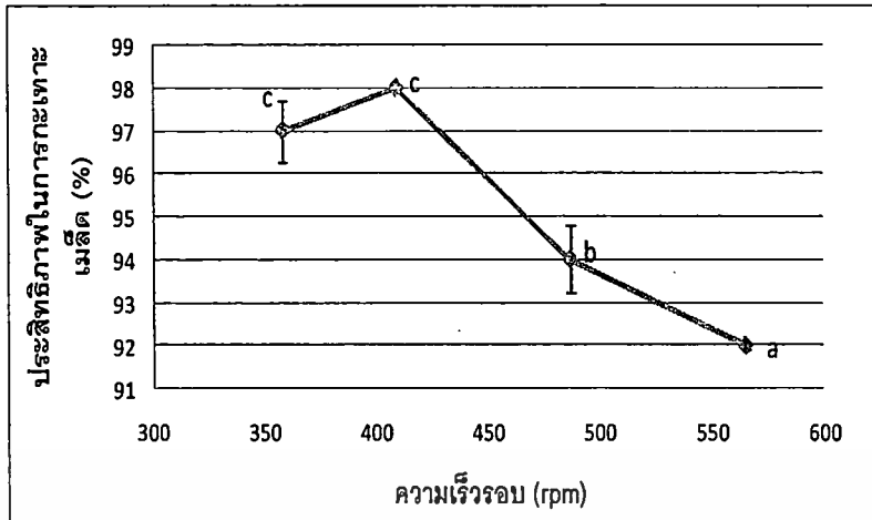
รูปที่ 4.9 ความสัมพันธ์ระหว่างความเร็วรอบและประสิทธิภาพในการกะเทาะเมทัลสบูดำ
