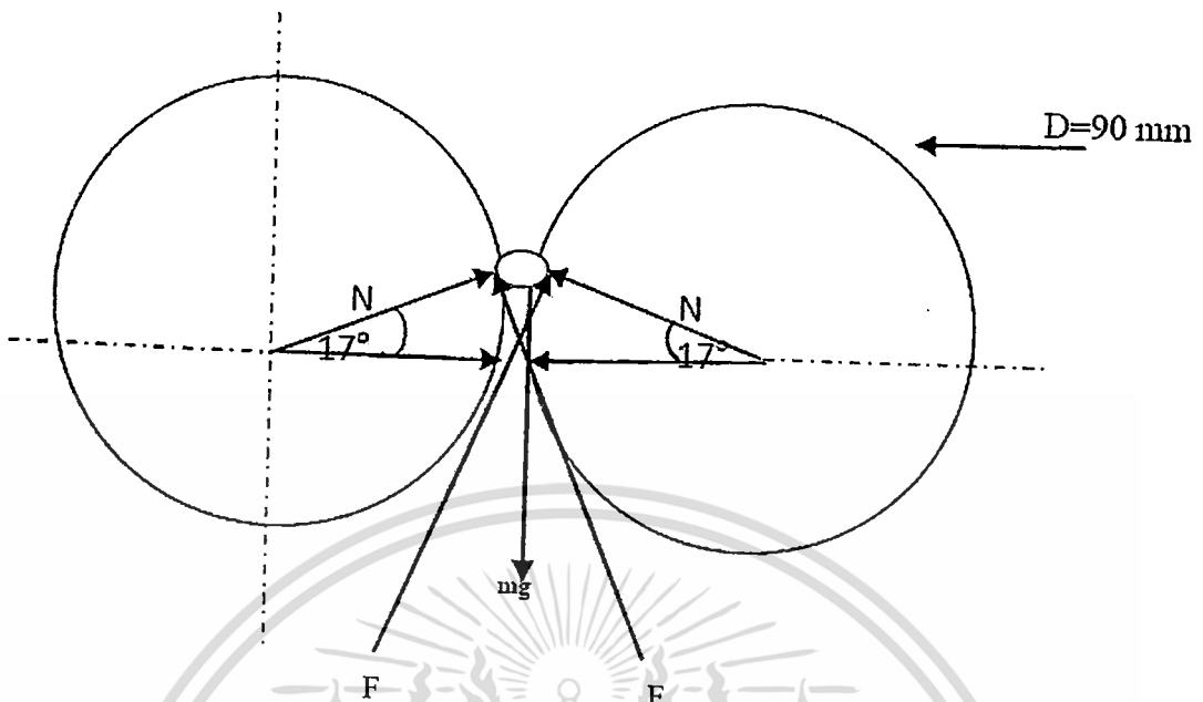
รูปที่ 3.6 ไตอะแกรมการรับแรงของเมตีดส์บู่ดำมีระยะห่างน้อยที่สุด 6 mm
