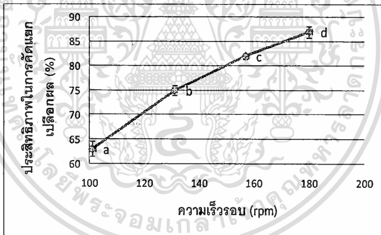
รูปที่ 4.8 ความสัมพันธ์ระหว่างความเร็วรอบและประสิทธิภาพในการตัดแยกเปลือกผล
