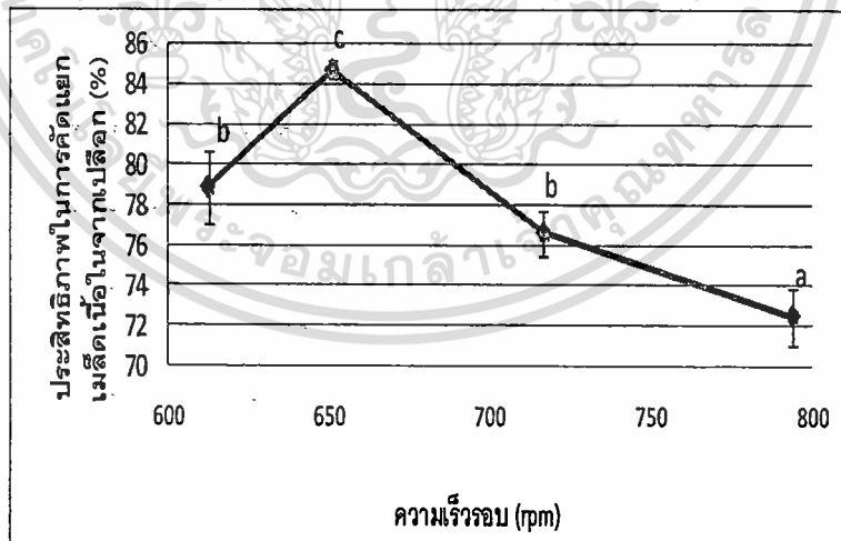
รูปที่ 4.12 ความสัมพันธ์ระหว่างความเร็วรอบและประสิทธิภาพในการคัดแยกเปลือกเมล็ดออกจากเนื้อในเมล็ด
