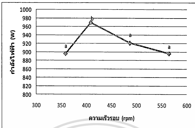
รูปที่ 4.11 ความสัมพันธ์ระหว่างความเร็วรอบและกำลังไฟฟ้าที่ใช้ในการกะเทาะเมล็ดสับดูดำ
