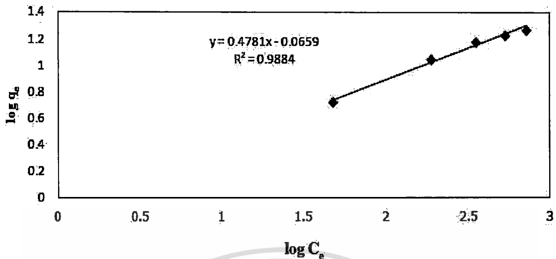
รูปที่ 9 ไอโซเทอมการดูดซับสารละลายสีย้อม RO16 ของ CHI-MMT 3 ซึ่งเป็นไอโซเทอมแบบฟรุนดลิช
