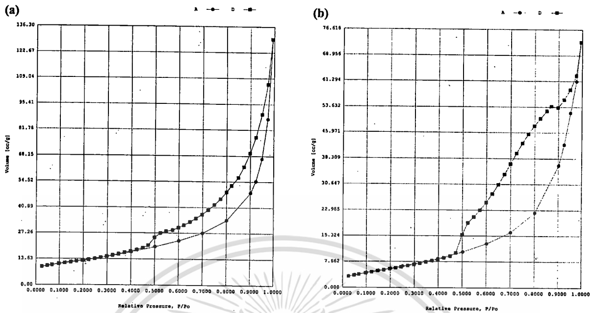
รูปที่ 5 ไอโซเทอมของการดูดซับและคายซับก๊าซใน โตรเจนของ (a) MMT และ (b) CHI-MMT 3
