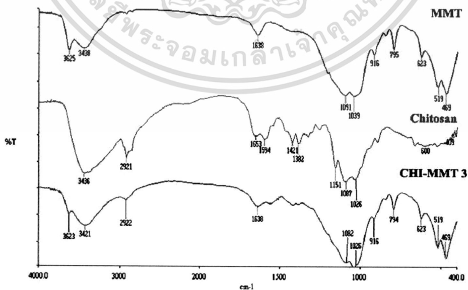
รูปที่ 4 อินฟราเรดสเปกตรัมของ MMT โคไคซาน และ CHI-MMT 3
