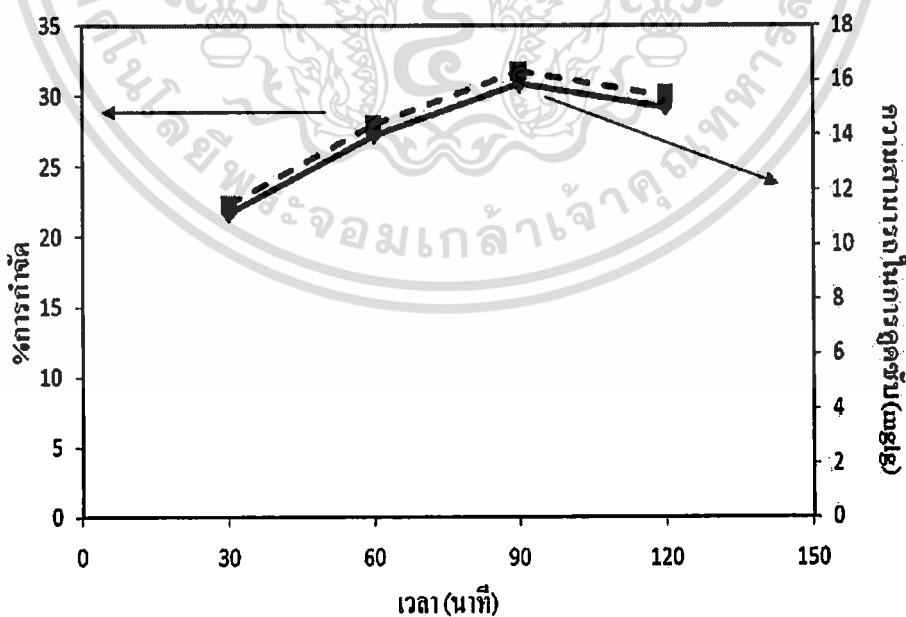
รูปที่ 7 กราฟแสดงความสัมพันธ์ระหว่าง%การกำจัดและความสามารถในการดูดซับของ CHI-MMT 3 กับระยะเวลาที่ใช้ในการดูดซับสารละลายสีย้อม RO16 โดยใช้ความเข้มข้นเริ่มต้นของสารละลายสีย้อมค่าคงที่เท่ากับ 500 มิลลิกรัม/ลิตร
