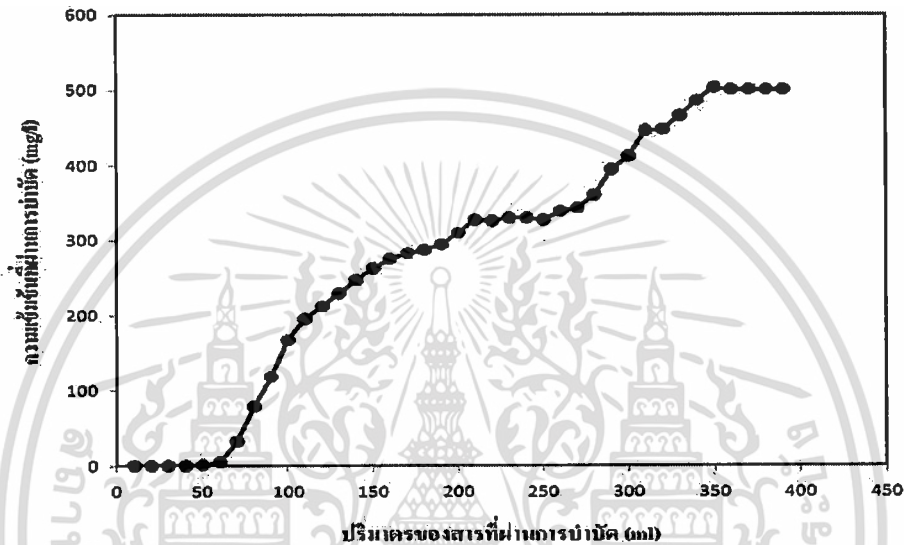
รูปที่ 11 กราฟแสดงความสัมพันธ์ระหว่างความเข้มข้นของสารละลายสีย้อม RO16 ที่ผ่านการบำบัดและปริมาตรสารที่ผ่านการบำบัด
