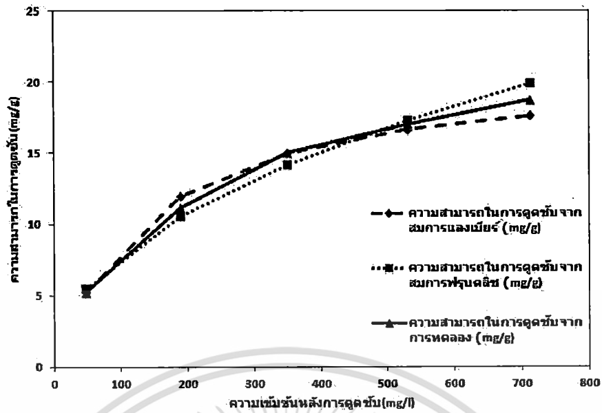
รูปที่ 10 กราฟแสดงความสามารถในการดูดซับที่ได้จากการทดลองจากสมการแมงเมียร์และสมการฟรุนดลิช
