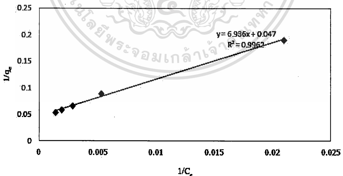
รูปที่ 8 ไอโซเทอมการดูดซับสารละลายสีย้อม RO16 ของ CHI-MMT 3 ซึ่งเป็นไอโซเทอมแบบแลงเมียร์
