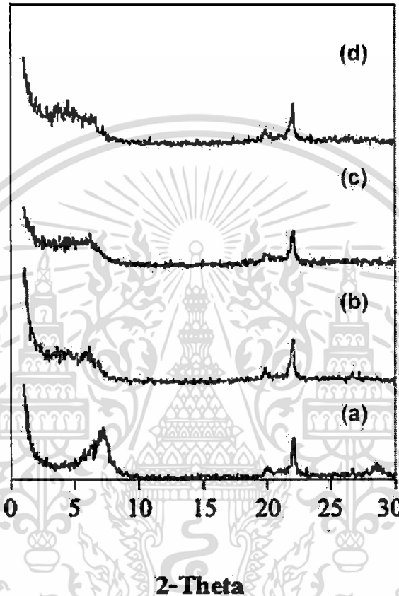
รูปที่ 2 รูปแบบการเลี้ยวเบนรังสีเอ็กซ์ของ (ก) MMT (ข) CHI-MMT 1 (ค) CHI-MMT 2 และ (ง) CHI-MMT 3
