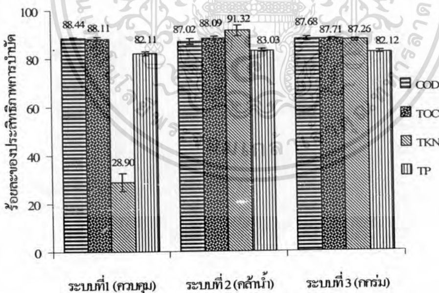
รูปที่ 4.2 การเปรียบเทียบประสิทธิภาพการกำจัดซีโอดี ทีเคเอ็น และฟอสเฟตทั้งหมดของระบบบึงประดิษฐ์แบบน้ำไหลได้ผิวดินแนวตั้งด้วยพืชต่างชนิดกัน
