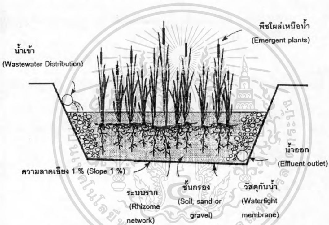
รูปที่ 2.3 ระบบบึงประดิษฐ์แบบน้ำไหลใต้ผิวดินแนวนอน (U.S.EPA, 2000(a))
