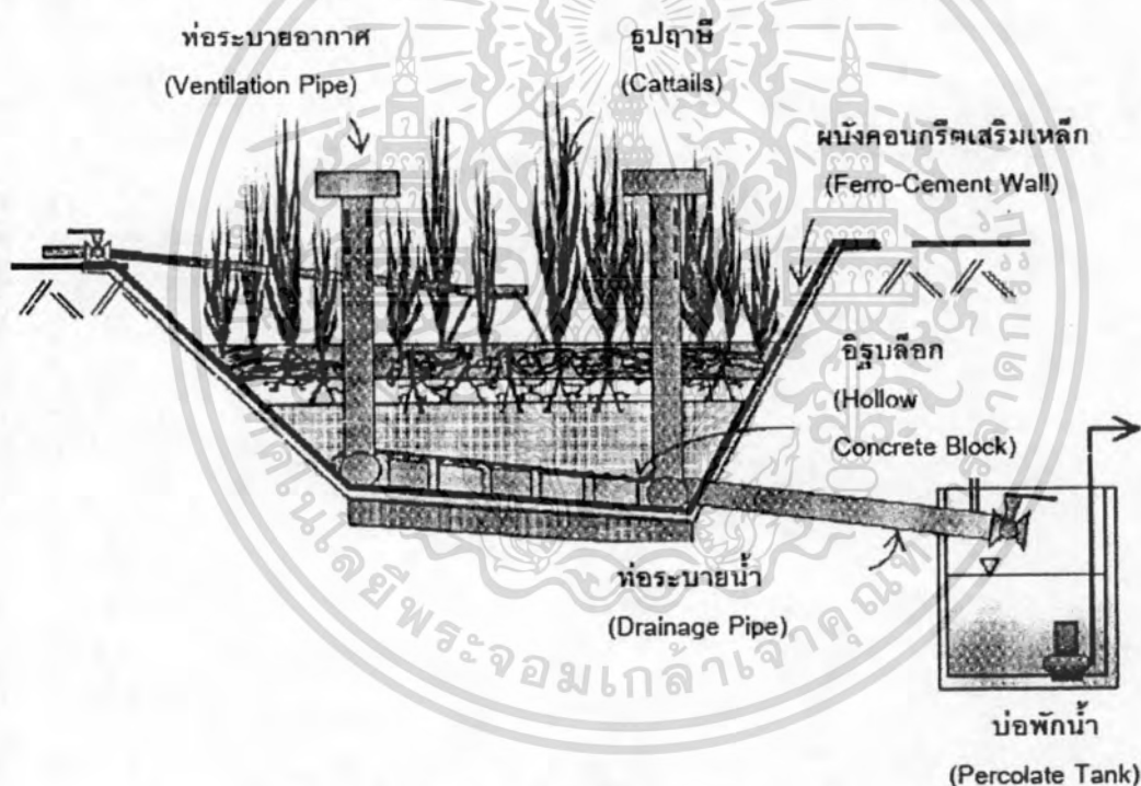
รูปที่ 2.4 ระบบบึงประดิษฐ์แบบน้ำไหลใต้ผิวดินแนวดิ่ง (U.S.EPA, 2000 (b))
