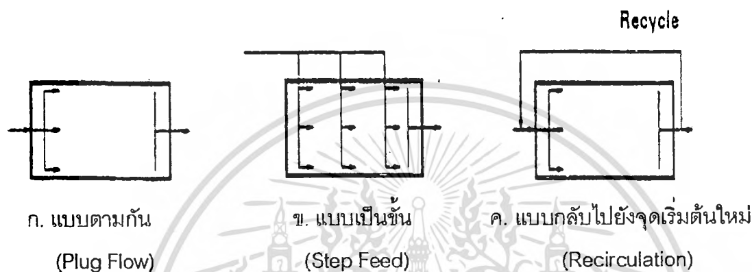
รูปที่ 2.5 รูปแบบการไหลของน้ำในบึงประดิษฐ์
