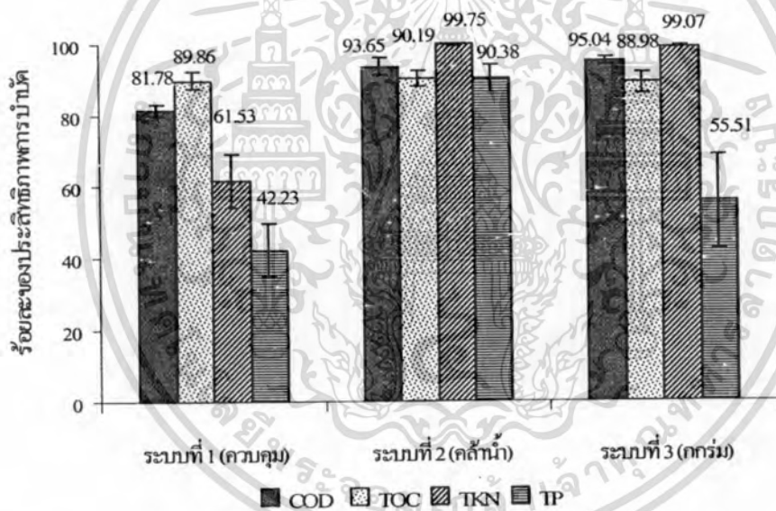
รูปที่ 4.7 การเปรียบเทียบประสิทธิภาพการกำจัดสารอินทรีย์คาร์บอน ที่เคเอ็น และฟอสเฟตทั้งหมด โดยใช้ระบบบึงประดิษฐ์แบบน้ำไหลได้ผิวดินแนวดิ่งในน้ำเสียชุมชนจากท่าอากาศยานสุวรรณภูมิ
