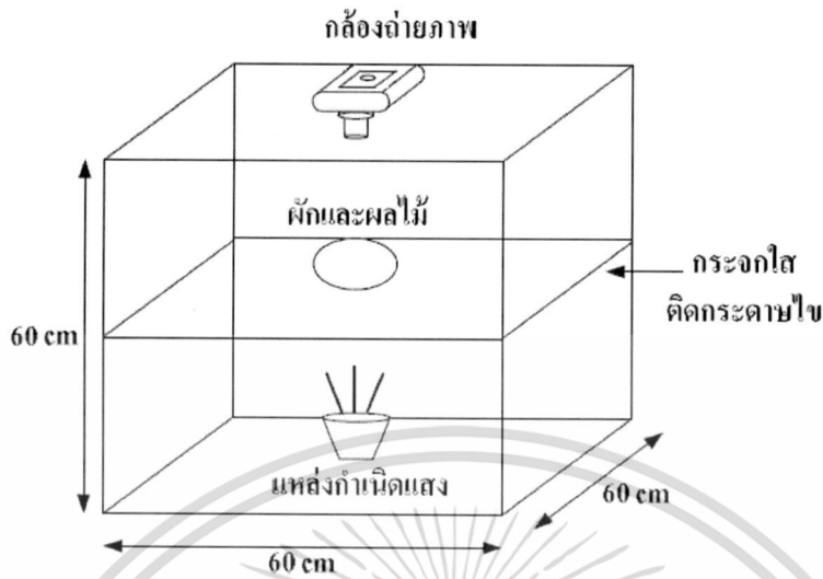
ภาพที่ 3.2 ส่วนประกอบของกล้องถ่ายภาพด้วยเทคนิคโฟลหลัง
