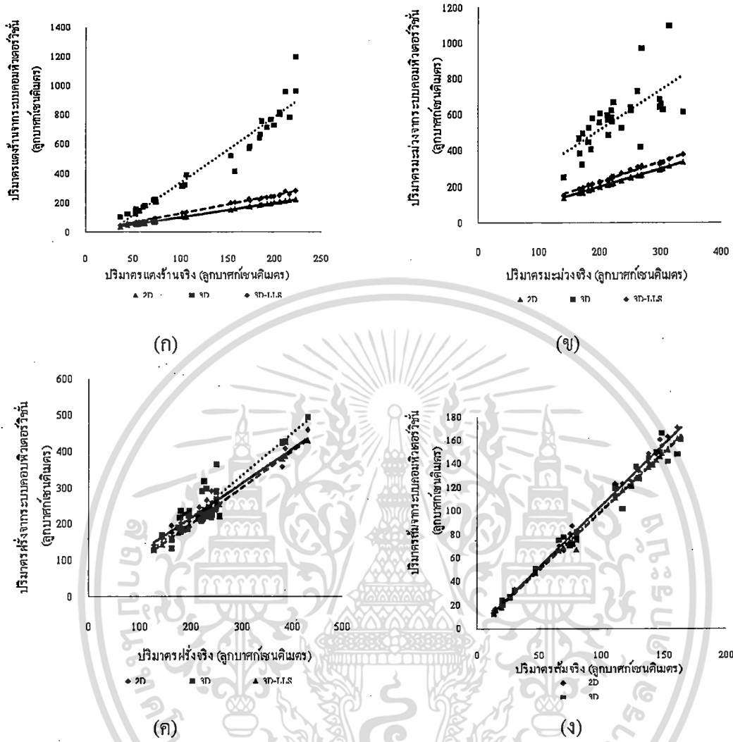
ภาพที่ 4.3 ความสัมพันธ์ระหว่างปริมาณจริงกับปริมาณจากระบบคอมพิวเตอร์วัดขึ้นทั้ง 3 เทคนิคของผักและผลไม้ชนิดต่างๆ
