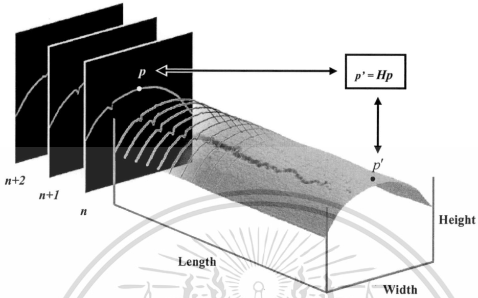
ภาพที่ 2.12 การประยุกต์ใช้ทฤษฎีโฮโมกราฟฟีในการตรวจวัดขนาดวัตถุ ที่มา : ศรายุทธ, 2553
