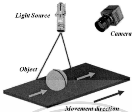
ภาพที่ 2.11 อุปกรณ์สำหรับเทคนิคการวัดขนาดวัตถุสามมิติโดยการใช้แสงเลเซอร์แบ่งส่วน ที่มา : ศรายุทธ, 2553
