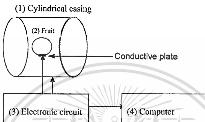
ภาพที่ 2.5 การวัดปริมาตรด้วยวิธีการวัดค่าความจุไฟฟ้า
