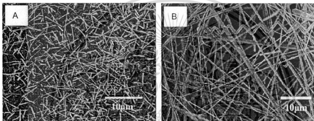
รูปที่ 2.17 แสดงลักษณะพื้นผิวที่มีเส้นลวดนาโนทินออกไซด์เกิดขึ้น
