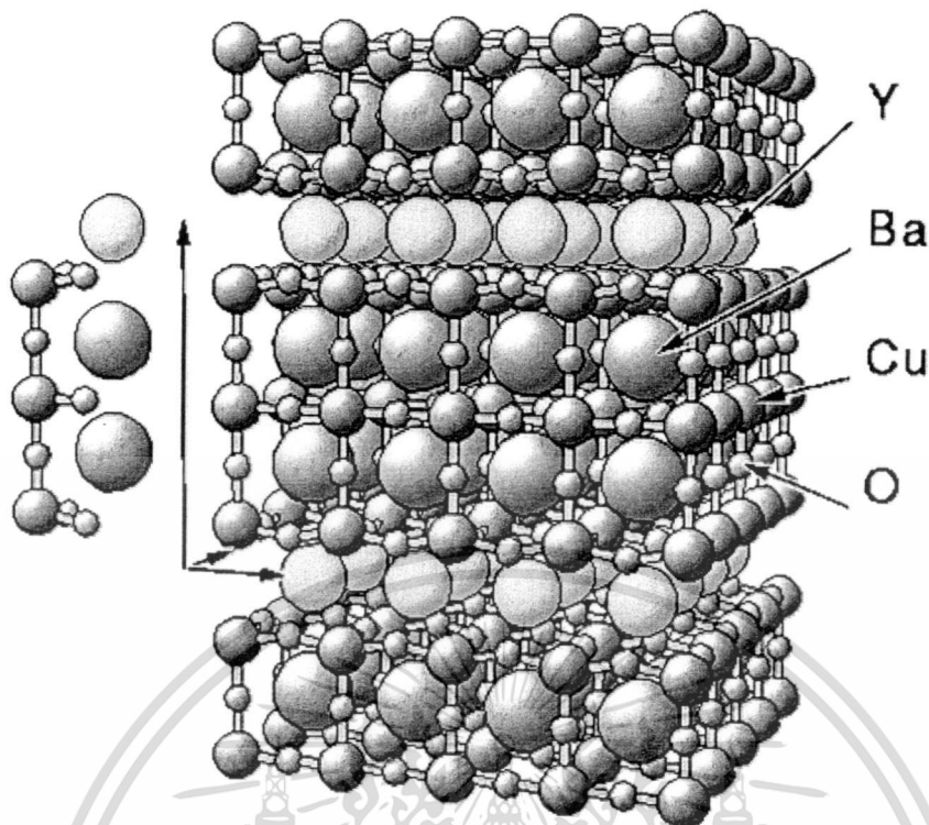
รูปที่ 2.8 โครงสร้างผลึกของตัวนำไฟฟ้ายิ่งยวด \text{YBa}_2\text{Cu}_3\text{O}_7 (.3) lattice ( www.fhi-berlin.mpg.de/th/personal/hermann/YBaCuO.gif )
