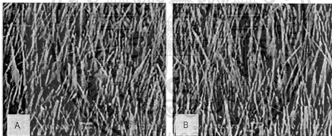
รูปที่ 2. 13 เส้นลวดนาโนคอปเปอร์ออกไซด์ A) เเผาที่อุณหภูมิ 500 องศาเซลเซียส และ B) เเผาที่อุณหภูมิ 600 องศาเซลเซียส (Huang 2004)
