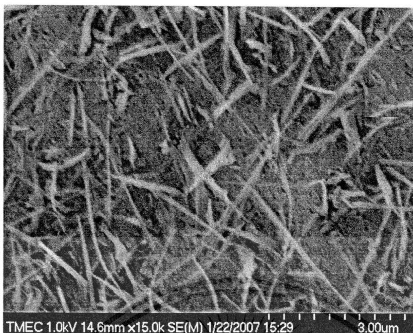
รูปที่ 4.10 เส้นลวดนาโนคอปเปอร์ออกไซด์ที่ได้จากการเผาในสภาวะออกซิเจน ที่อุณหภูมิ 550 องศาเซลเซียส 4 ชั่วโมง
