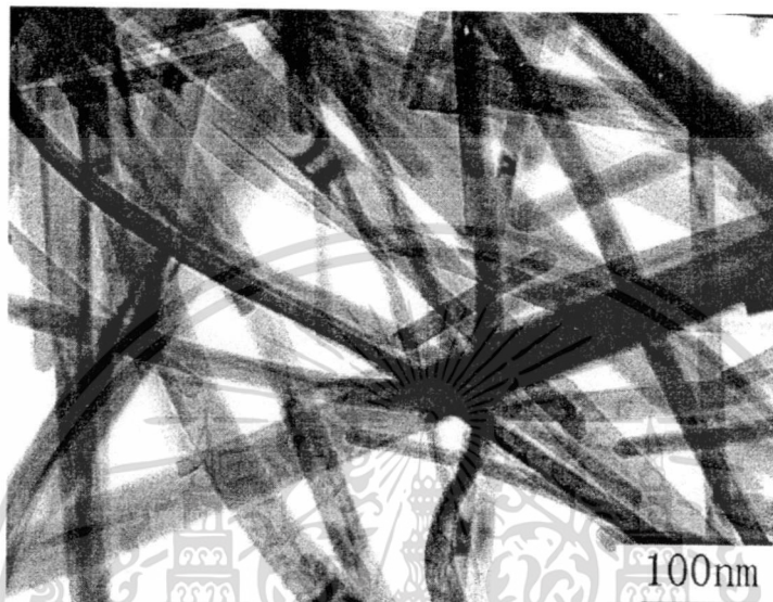
รูปที่ 2.9 แท่งนาโนซิงค์ออกไซด์ (ZnO nanorods) (Xu 2002)
