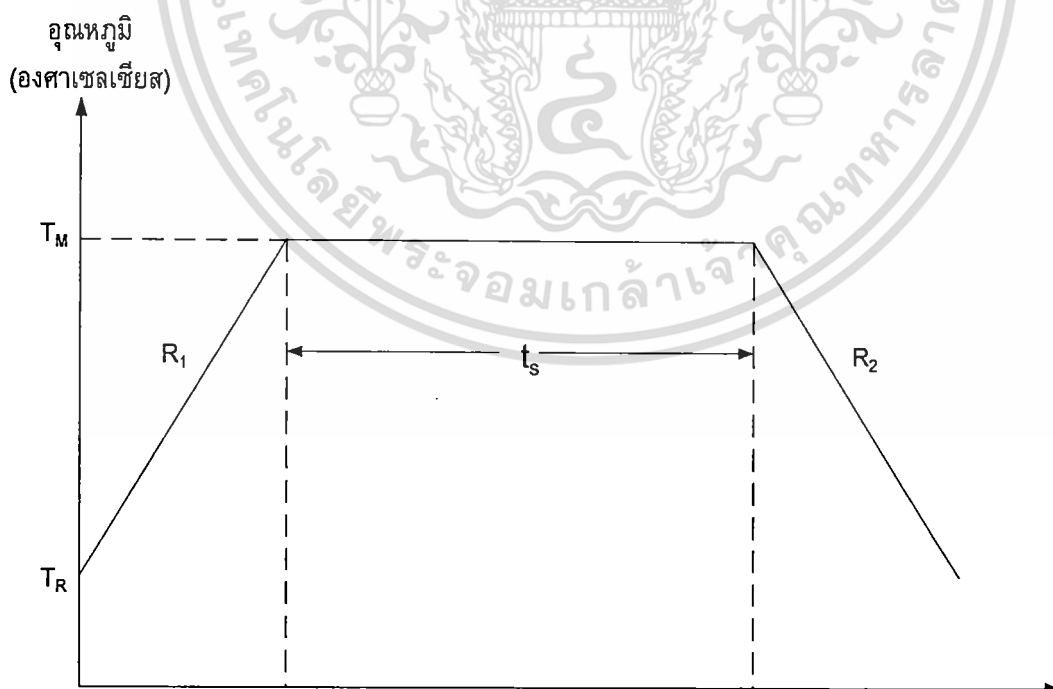
รูปที่ 3.2 แผนผังการเผาแคลไซน์ของแผ่นคอปเปอร์
