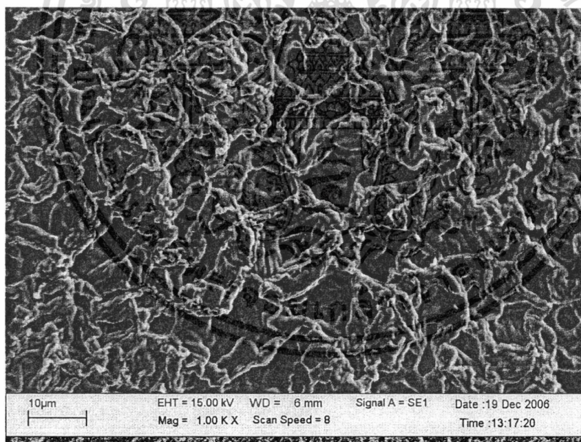
รูปที่ 4.11 ลักษณะของแผ่นคอปเปอร์ที่ได้จากการเผาในสภาวะออกซิเจน ที่อุณหภูมิ 700 องศาเซลเซียส 4 ชั่วโมง
