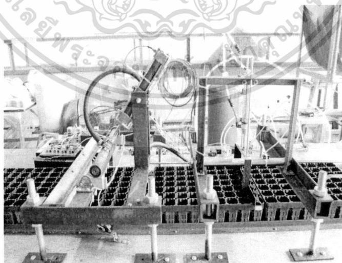
รูปที่ 3.1 เครื่องหยอดเมล็ดพืชลงถาดเพาะกล้าต้นแบบ
