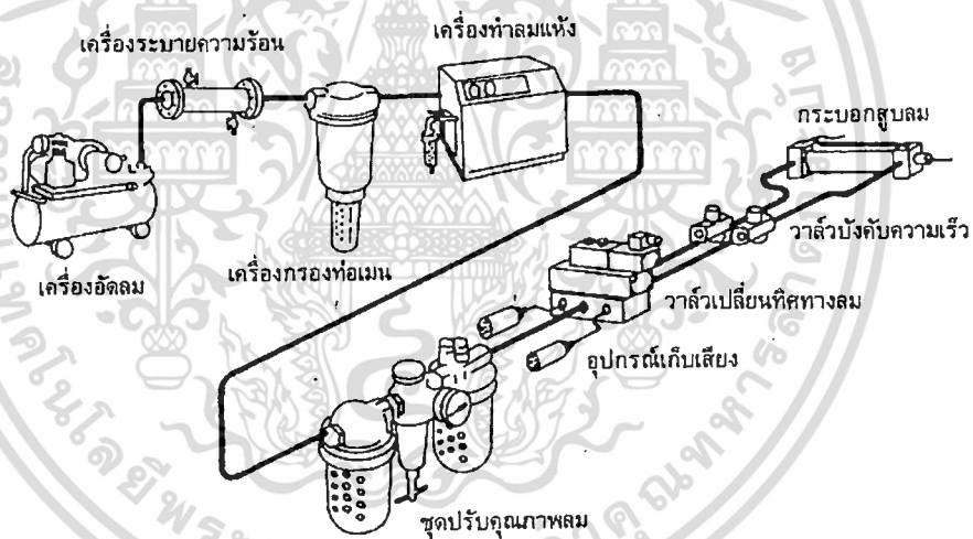
รูปที่ 2.16 อุปกรณ์และระบบนิวเมติก
