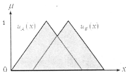
รูปที่ 2.3 แสดง A \cup B
