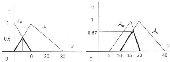
รูปที่ 2.7 แสดงการหาค่าน้ำหนัก w_1
