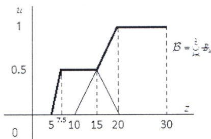
รูปที่ 2.11 แผนภาพแสดงการทำ B = \bigcup_{k=1}^2 B_k
