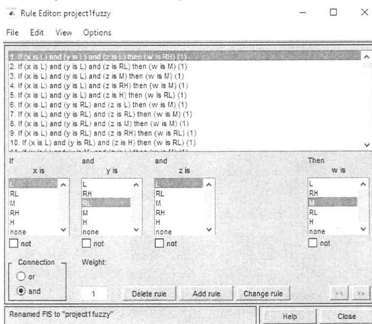
รูปที่ 5.1 แสดงนำเข้าข้อมูลสำหรับการกำหนดกฎฟuzzy
