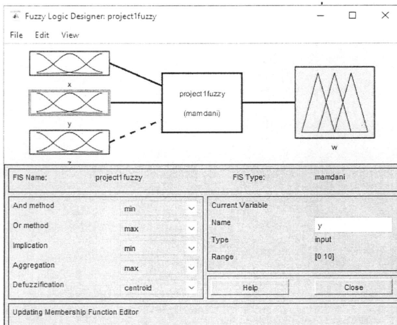
รูปที่ 5.1 แสดงนำเข้าข้อมูลสำหรับการกำหนดกฎฟuzzy
