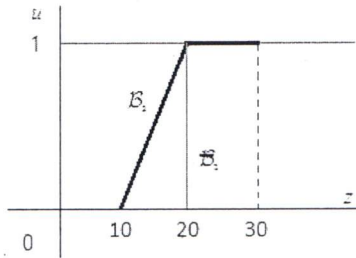
รูปที่ 2.10 แสดงการตัดยอด B_2 ด้วย w_2
