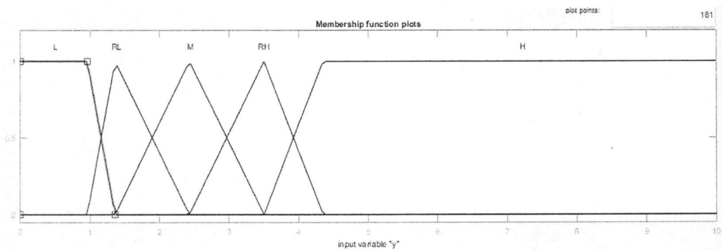
รูปที่ 4.3 แสดงเซตฟัซซีของตัวแปรภาษา P/BV
