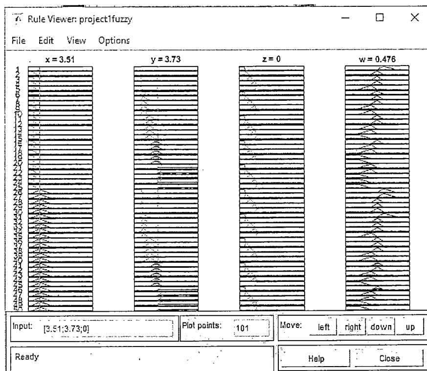
รูปที่ 5.3 แสดงแผนภาพกฎฟuzzyในการอนุมานด้วยวิธีแมมดานี
