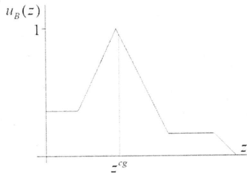
รูปที่ 2.12 แสดงเอาท์พุตค่าดั้งเดิม z^{cg} ด้วยวิธีจุดศูนย์กลางถ่วง
