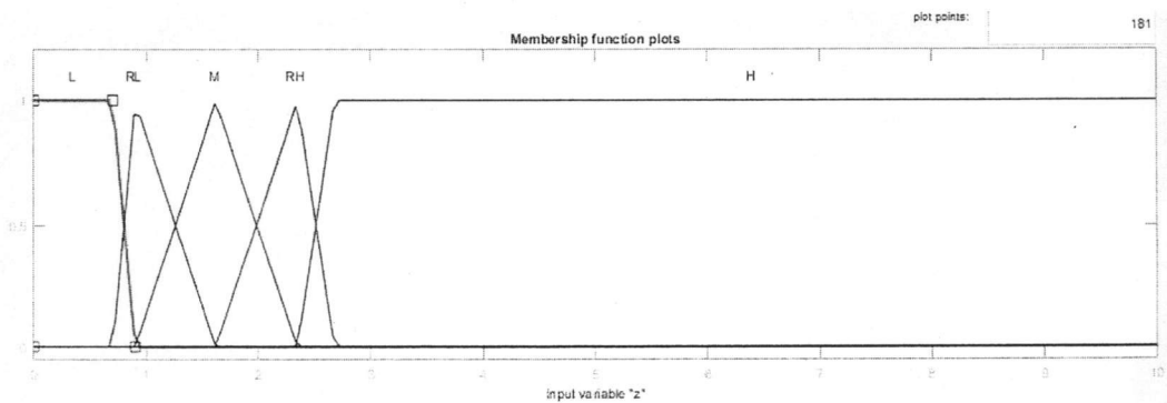
รูปที่ 4.4 แสดงเซตฟัซซีของตัวแปรภาษา P/Pn
