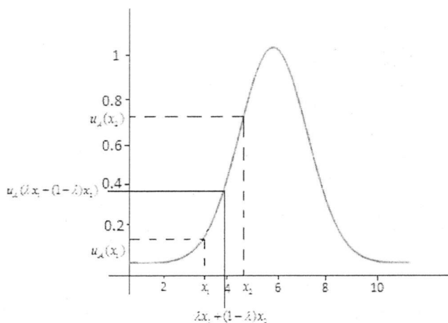
รูปที่ 2.4 แสดงเซตฟuzzy
