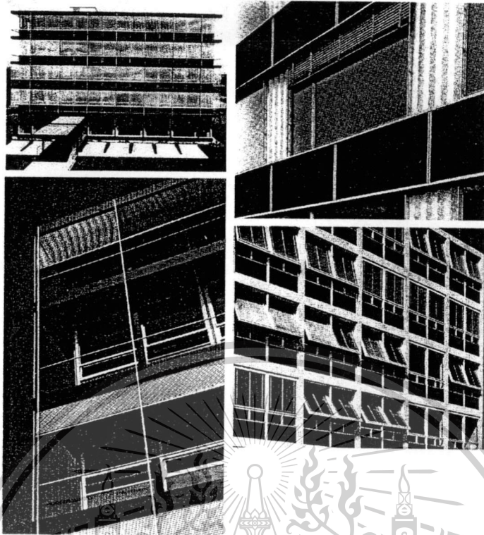
รูปที่ 2.16 ม่านบังแดด (Blinds) สำหรับภายนอกอาคาร ที่มา: Danz, Ernst. (1967)
