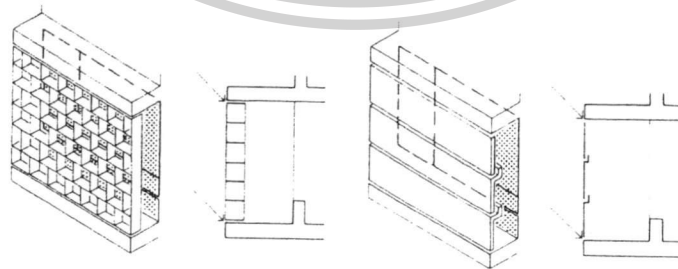
รูปที่ 2.23 ฉนวนสกรีนเพื่อการบังแดด
