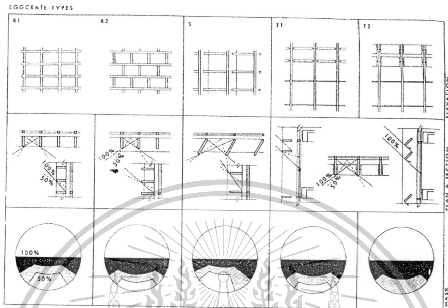
รูปที่ 2.29 แผงบังแดดแบบผสมหรือแบบรังไข่ (Eggcrate) (R) แผงบังแดดแบบผสม มีทั้งอุปกรณ์บังแดดแนวตั้งและแนวนอนจึงให้ลักษณะการบังแดดที่หลากหลาย (S) แผงบังแดดแบบผสมแบบทึบที่มีอุปกรณ์บังแดดทางตั้ง (T1) แผงบังแดดแบบผสมที่มีอุปกรณ์บังแดดแนวนอนแบบปรับได้ จะมีลักษณะการบังแดดแตกต่างไปตามการปรับมุม (T2) แผงบังแดดแบบผสมที่มีอุปกรณ์บังแดดแนวนอนแบบปรับได้ทั้งหมด 45 องศา
