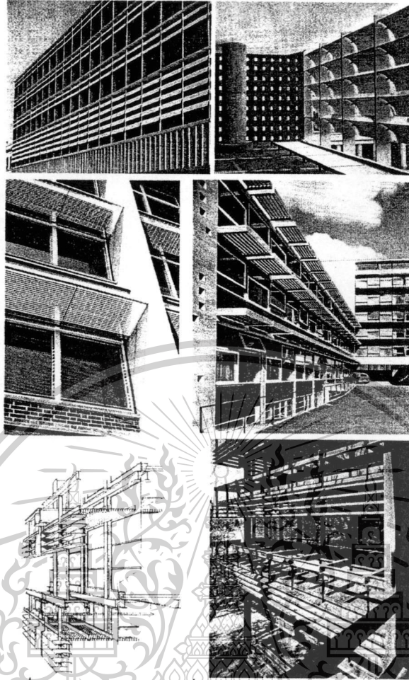
รูปที่ 2.14 เกล็ดบังแดดที่มีการออกแบบใช้กับอาคาร ที่มา: Danz, Ernst. (1967)
