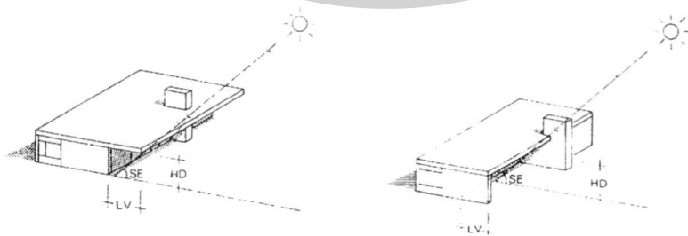
รูปที่ 2.4 การบังแดดในมุมสูงและสามารถกันลมแรงด้วยผนังด้านข้าง (HD คือความสูงของหลังคา LV คือ ระยะเวลาของหลังคา SE คือ มุมของดวงอาทิตย์)
