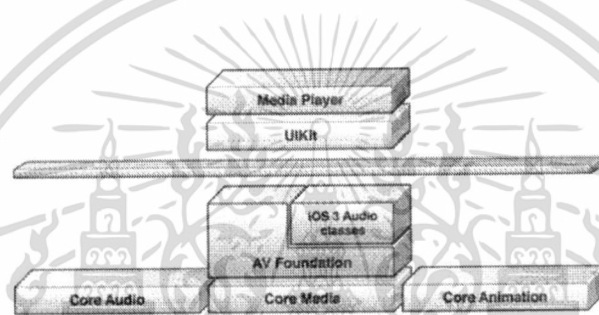
รูปที่ 2.12 Media Layer Hierarchy
