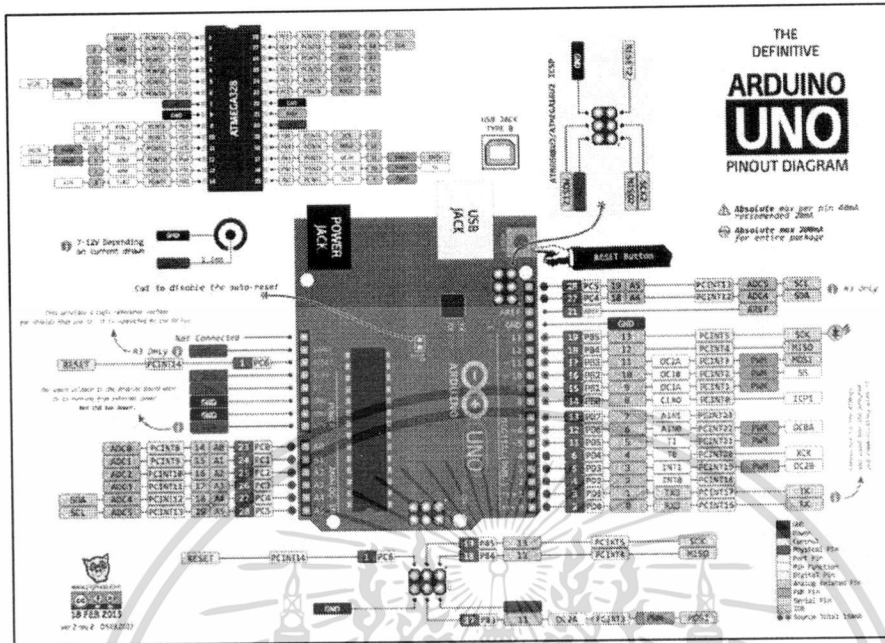
รูปที่ 2.13 Diagram ตำแหน่งขาพอร์ตไมโครคอนโทรลเลอร์ Arduino Uno R3
