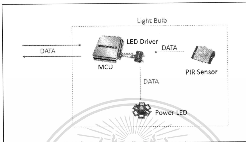
รูปที่ 3.14 แผนผังส่วนประกอบของหลอดไฟ
