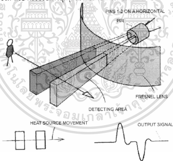
รูปที่ 2.7 การทำงานของเซ็นเซอร์จับความเคลื่อนไหว
