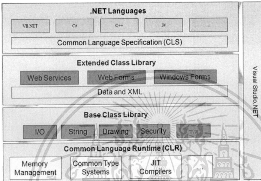
รูปที่ 2.4 แสดงสถาปัตยกรรมของโปรแกรม Microsoft Visual Studio 2008 เปรียบเทียบการทำงานของ .NET กับ JAVA
