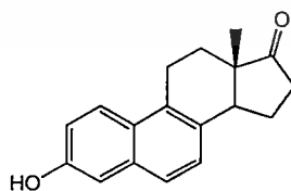
Equilenin (9)
