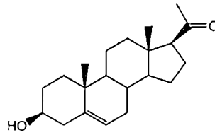
Pregnenolone (1)
