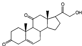
Cortisone (7)
