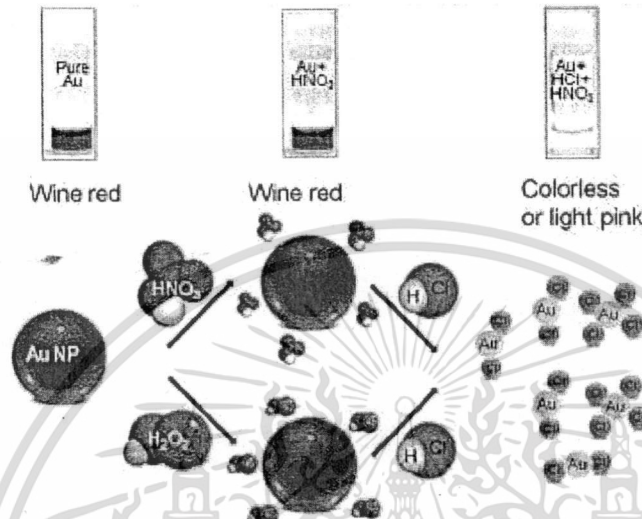
รูปที่ 2.2 แสดงกลไกในการเปลี่ยนแปลงสีของ AuNPs เมื่อมีและไม่มี HCl และ oxidizer
