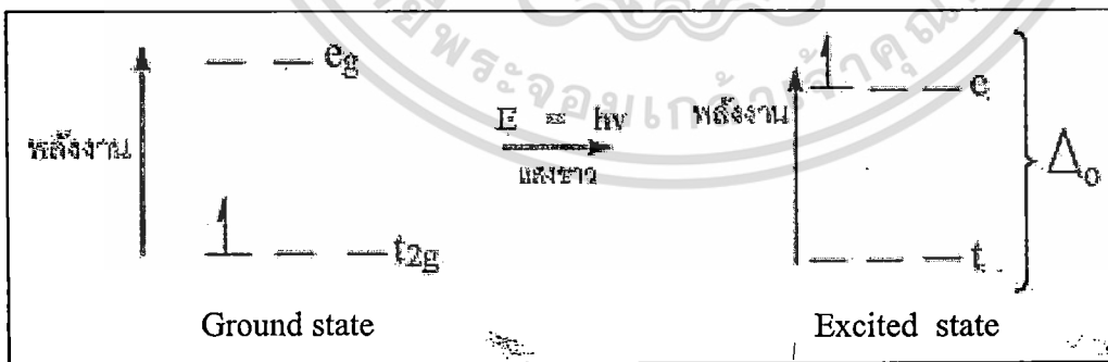
รูปที่ 2.4 การบรรจุอิเล็กตรอนของ Ti^{3+} ใน 3d-orbital ซึ่งมีโครงสร้างแบบ octahedral
