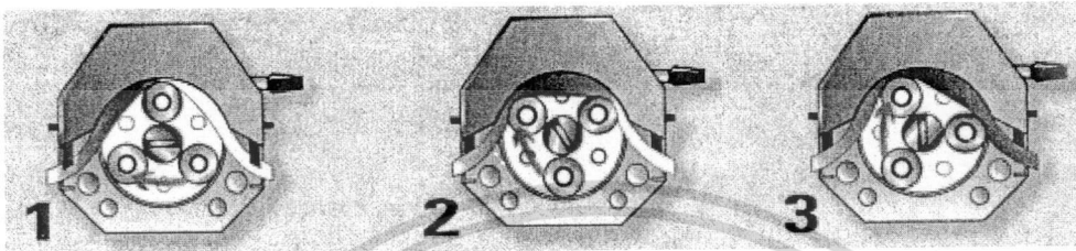
รูปที่ 2.8 แสดงการทำงานของ Peristaltic pump
