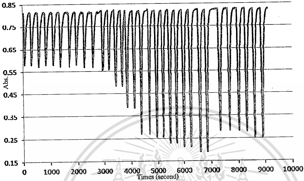
รูปที่ 4.12 แสดงสัญญาณที่ได้จากการวิเคราะห์ด้วยระบบ FIA ที่พัฒนาขึ้น โดย 10 พีคแรกเป็นสัญญาณของเบลงค์ 16 พีคต่อมาเป็นสัญญาณของสารละลายมาตรฐาน H_2O_2 ความเข้มข้น 0.5, 1, 2.5, 5, 10, 12.5, 15, 17.5 และ 20 ppm ความเข้มข้นละ 2 พีค และ 6 พีคสุดท้ายเป็นสัญญาณของตัวอย่างยา และผลิตภัณฑ์ซักผ้าขาว 2 ตัวอย่าง ตัวอย่างละ 2 ซ้ำ
