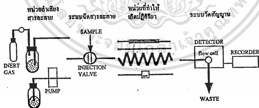
รูปที่ 2.7 แสดงส่วนประกอบของระบบ FIA
