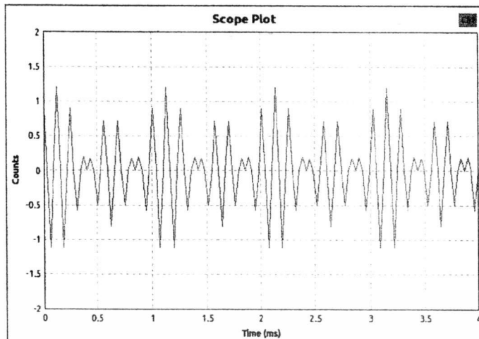
ภาพที่ 4.19 สัญญาณ เมื่อมีค่ามอดูเลชันอินเด็กซ์เท่ากับ 2
