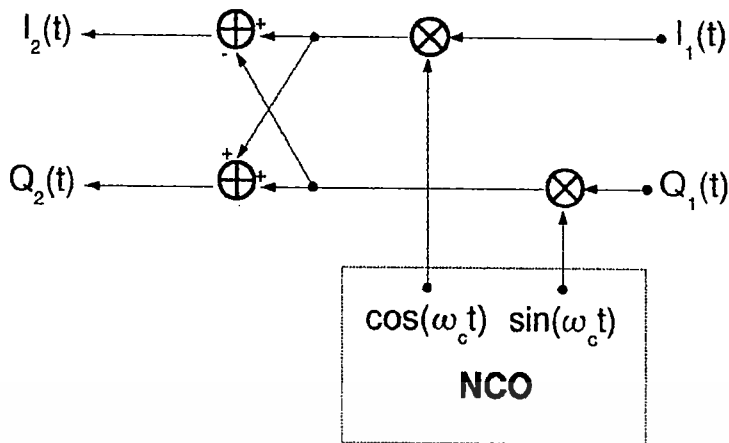
ภาพที่ 2.6 Digital Up-Conversion (DUC) ใน USRP
