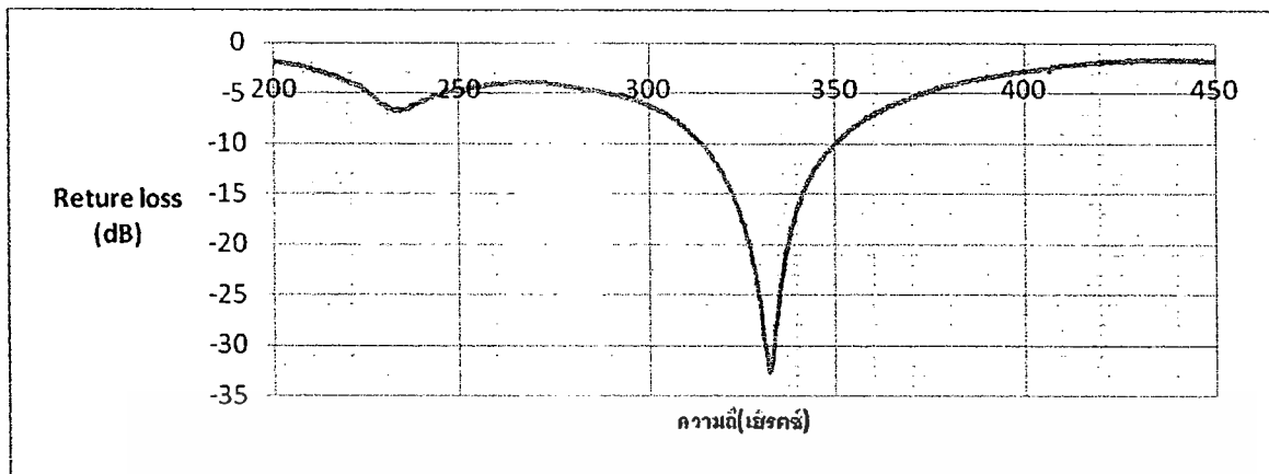
ภาพที่ 4.4 กราฟ Return loss ที่ความถี่ 329.6 MHz
