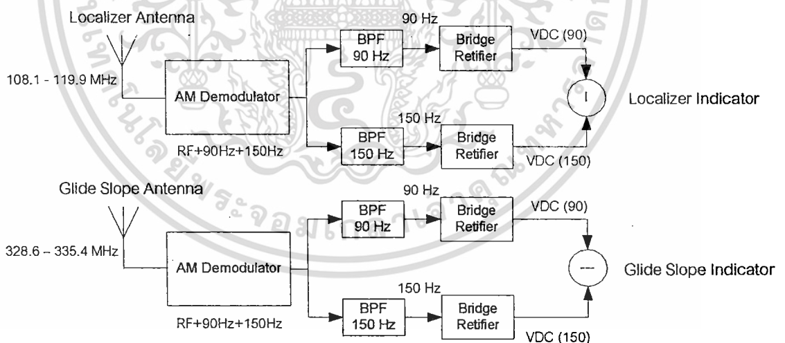
ภาพที่ 2.11 บล็อกไดอะแกรมการทำงานของเครื่องรับ ILS แบบอนาล็อก
