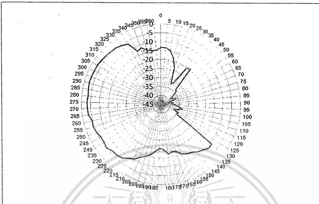
ภาพที่ 4.9 Cross H plane 329.6 MHz
