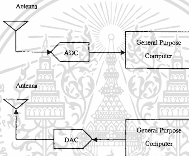
ภาพที่ 2.1 บล็อกไดอะแกรม ระบบวิทยุควบคุมโดยซอฟต์แวร์
