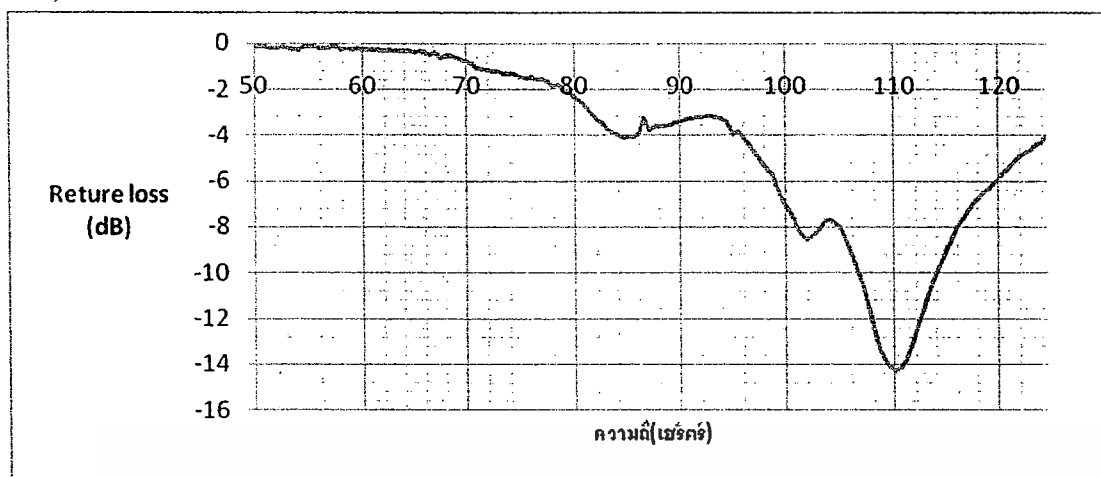
ภาพที่ 4.2 กราฟ Return loss ที่ความถี่ 110 MHz
