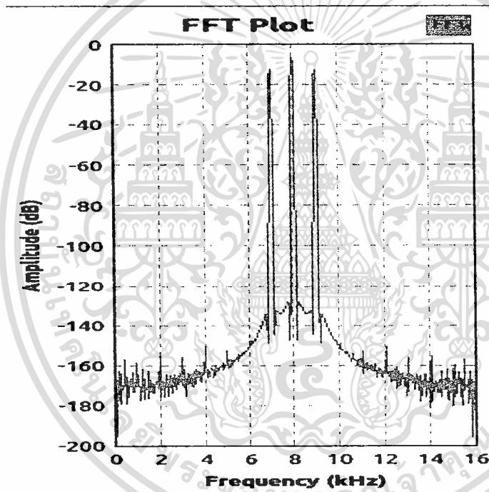
ภาพที่ 4.14 สเปกตรัมสัญญาณเมื่อมีค่ามอดูเลชันอินเดกซ์เท่ากับ 1
