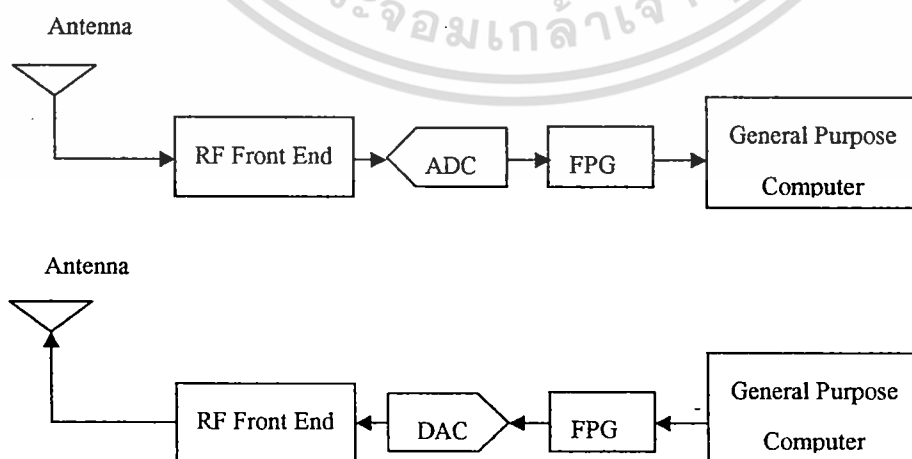
ภาพที่ 2.2 บล็อกไดอะแกรมการใช้งานระบบการสื่อสารแบบ SDR ในปัจจุบัน
