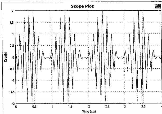
ภาพที่ 4.15 สัญญาณเมื่อมีค่ามอดูเลตชันอินเด็กซ์เท่ากับ 1
