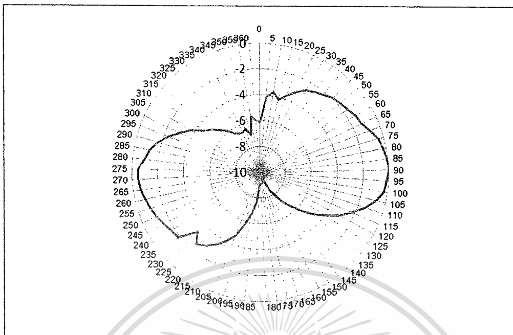
ภาพที่ 4.5 Co-H plane ที่ความถี่ 110.5 MHz
