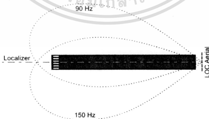
ภาพที่ 2.8 ลักษณะการแพร่กระจายคลื่นของสถานี Localizer
