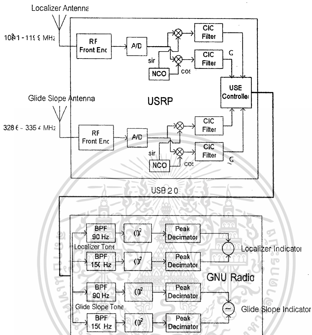
ภาพที่ 3.2 แผนผังการทำงานของระบบส่วนของ USRP และ GNU Radio
