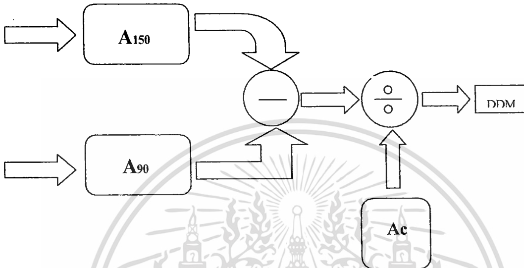
ภาพที่ 3.14 แผนผังการทำงานเพื่อหาค่า DDM
