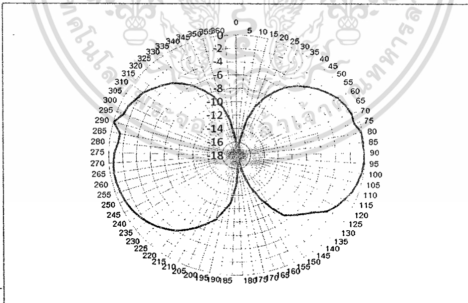
ภาพที่ 4.8 Co-H plane 329.6 MHz
