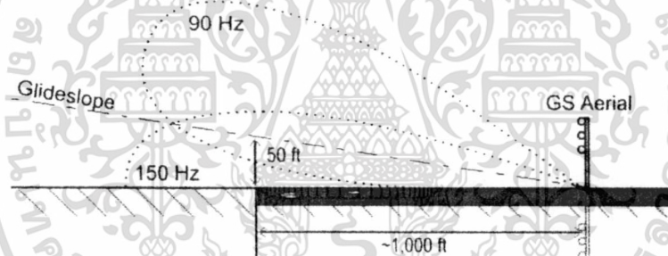
ภาพที่ 2.9 ลักษณะการแพร่กระจายคลื่นของสถานี Glide Slope
