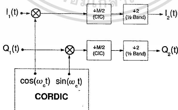
ภาพที่ 2.5 Digital Down Conversion (DDC) ใน USRP
