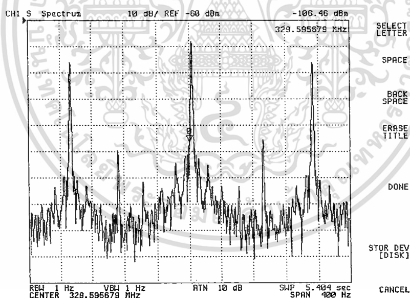
ภาพที่ 4.3 สัญญาณในย่าน Glide slope
